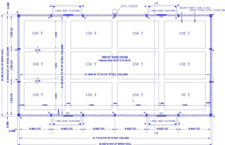
PLAN FOR 1/1800 MT.
